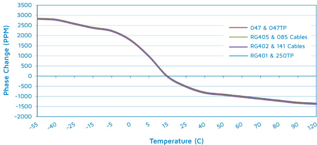
Phase vs. Temperature (°C)
