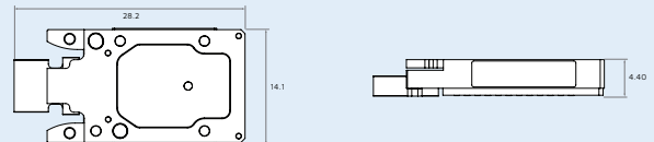
Actual size of LightABLE 28G LL 4TRX*
